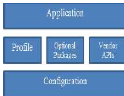
Gambar 1. Arsitektur J2ME
