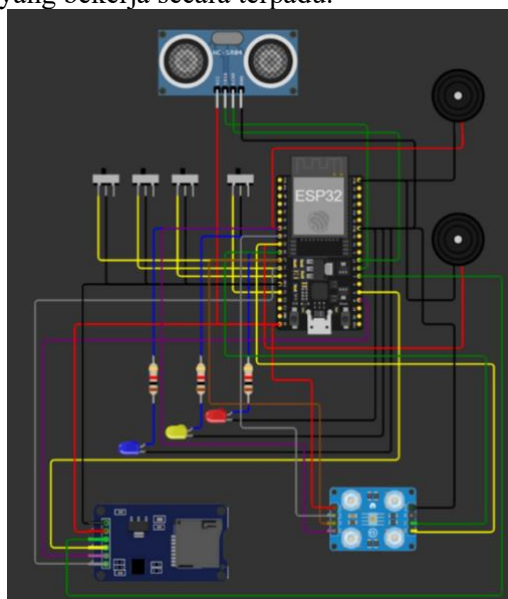
Gambar 4 Perancangan Perangkat Keras
