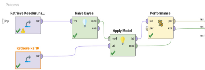
Gambar 19. Proses Pengujian Confusion Matrix dengan data testing 10% dari keseluruhan responden
